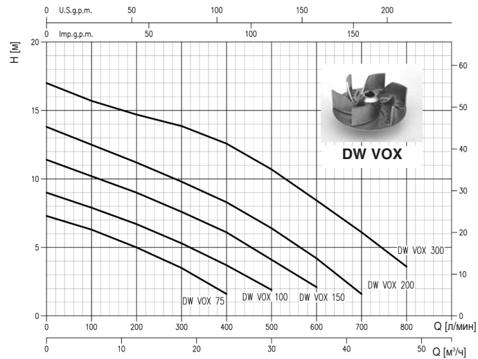
Со спуском и соединительной опорой
